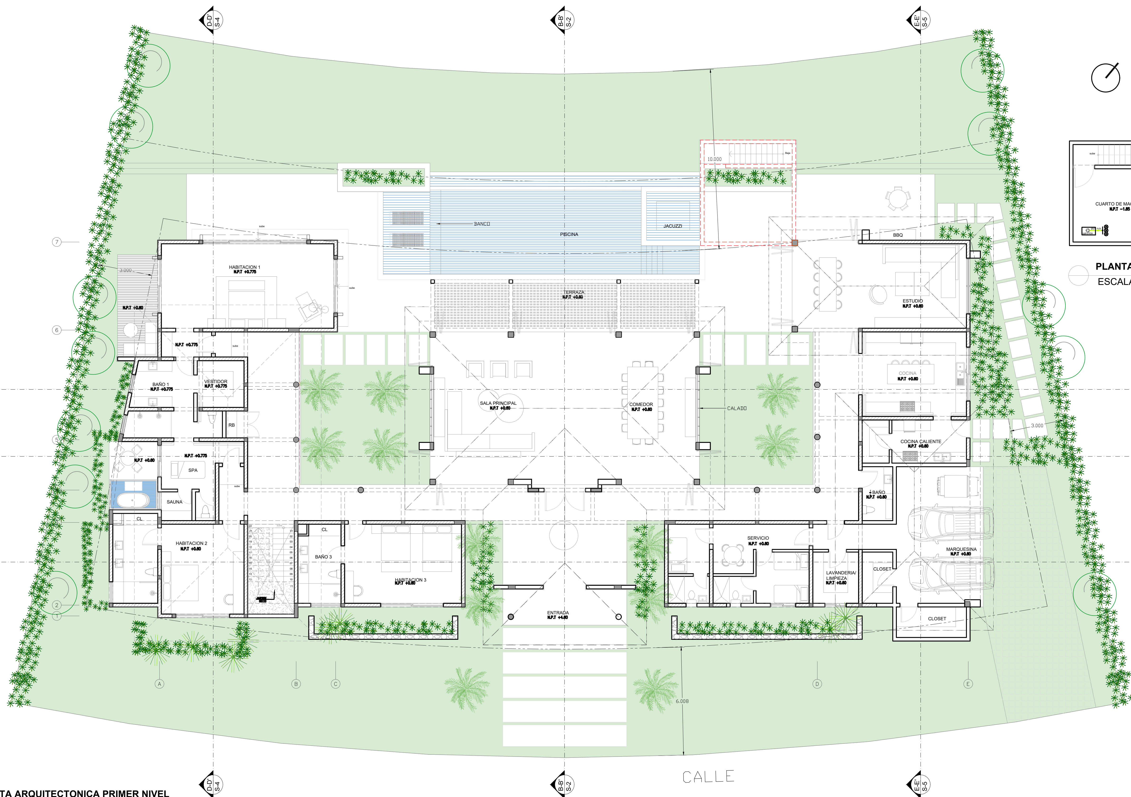
PLANTA ARQUITECTONICA PRIMER NIVEL ESCALA: 1:100
