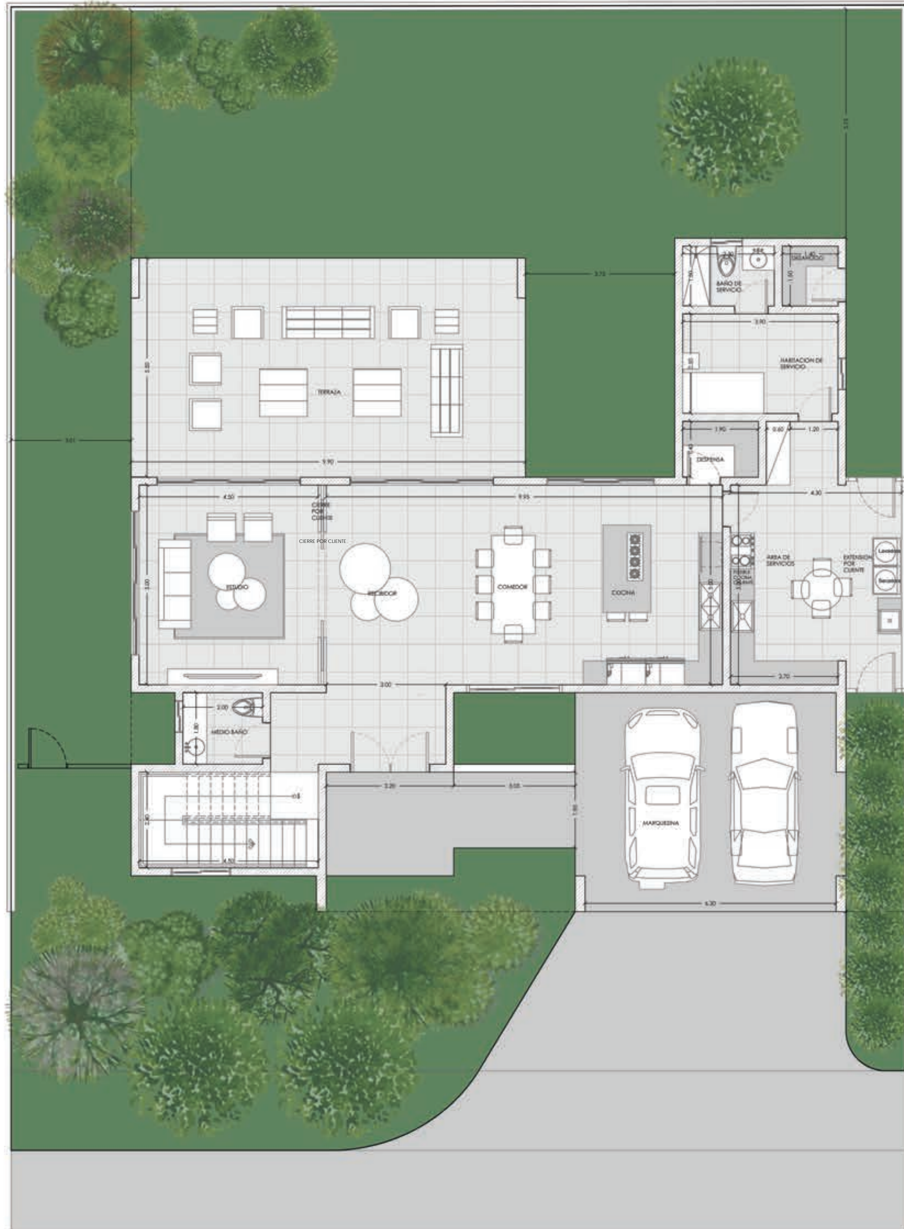
Planta Arquitectónica Nivel 1
