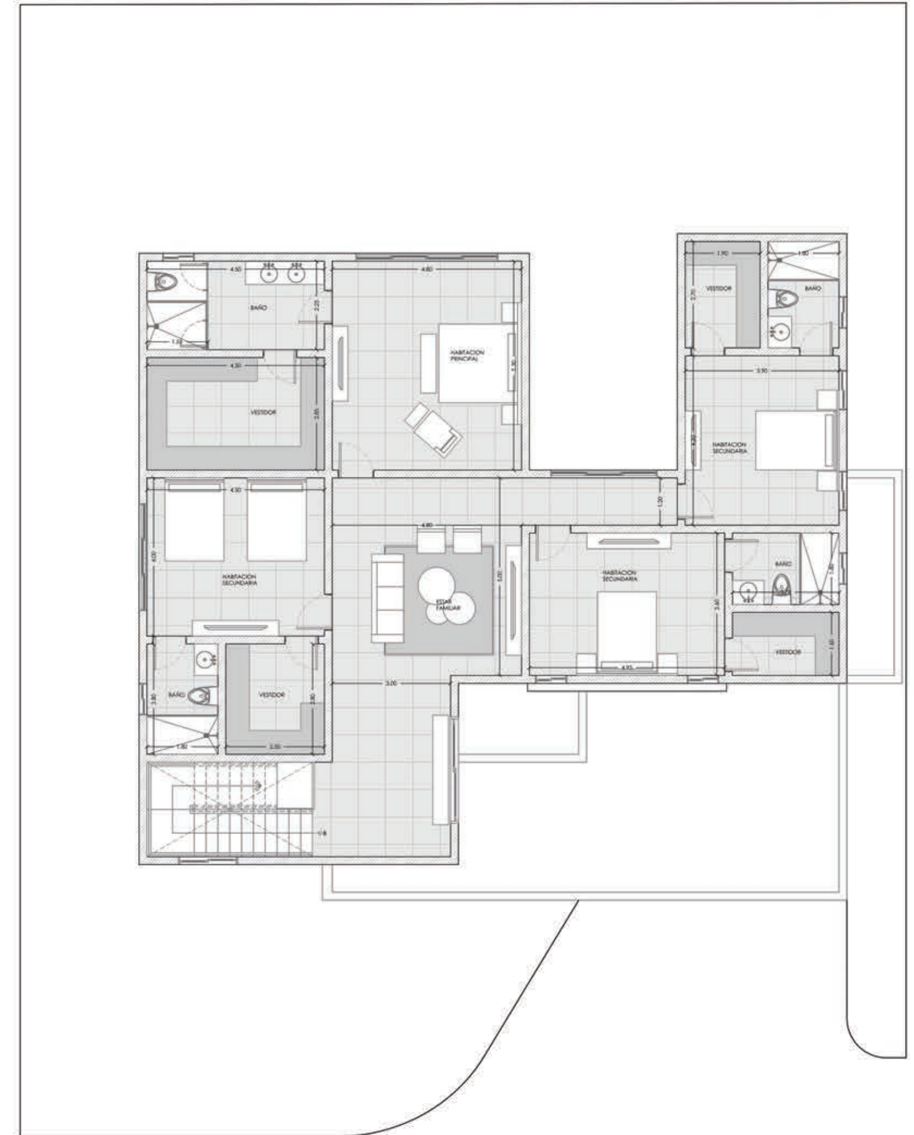
Planta Arquitectónica Nivel 2
