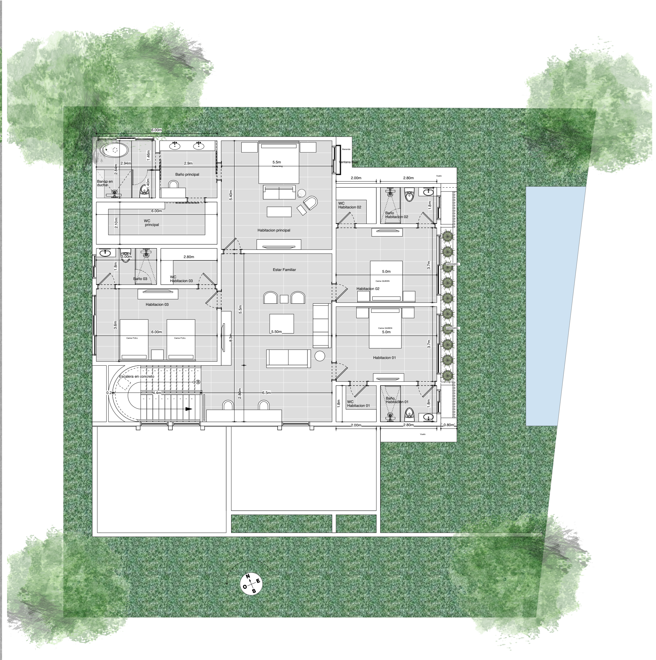
Planta Arquitectónica Nivel 2
