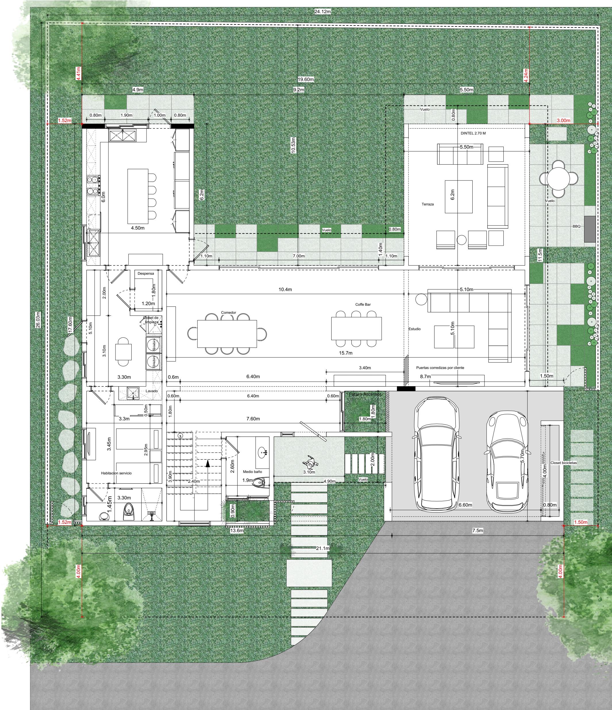
Planta Arquitectónica Nivel 1
