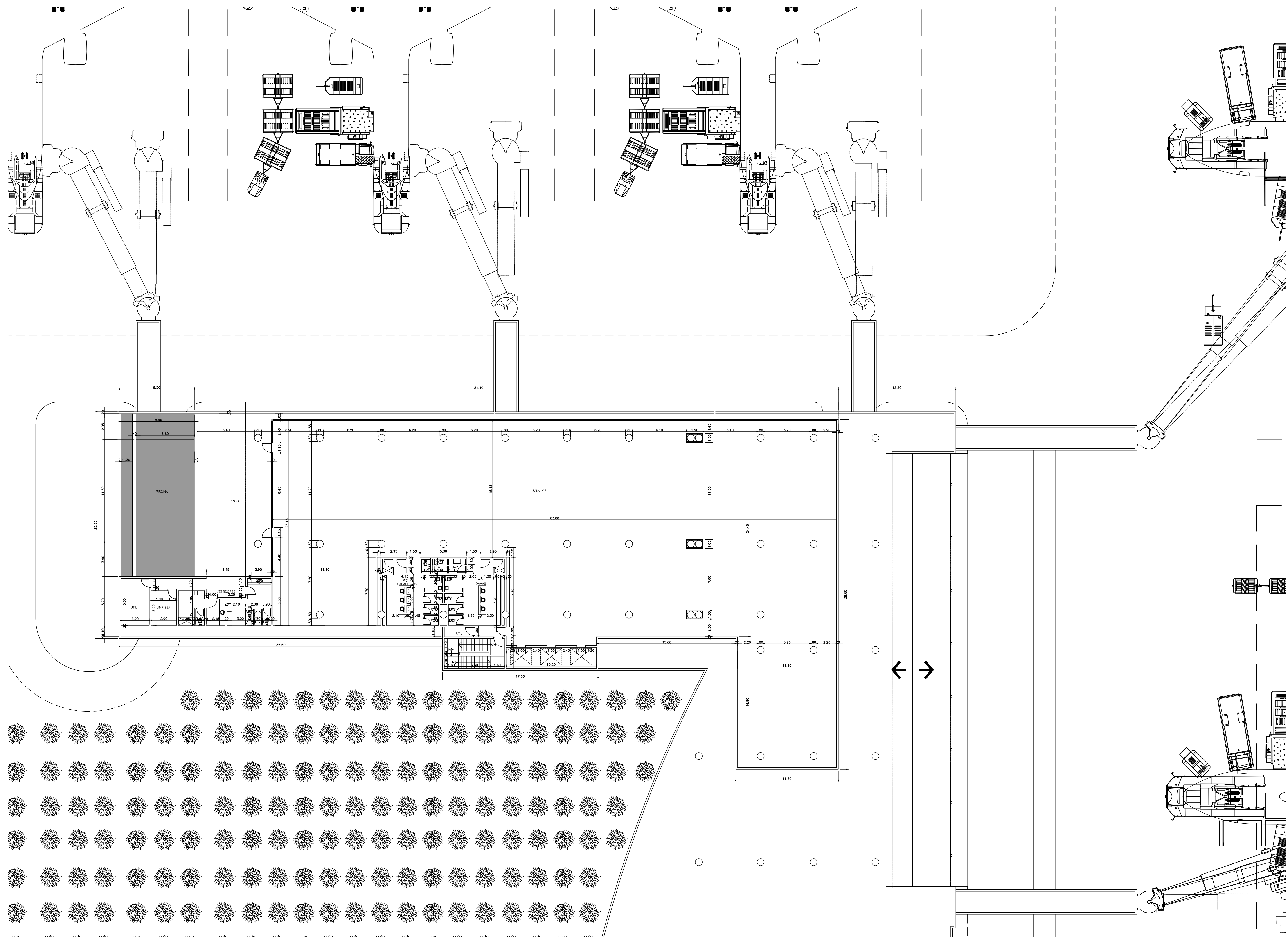
TERMINAL B2 - PLANTA DE VIP ESCALA: 1:200
