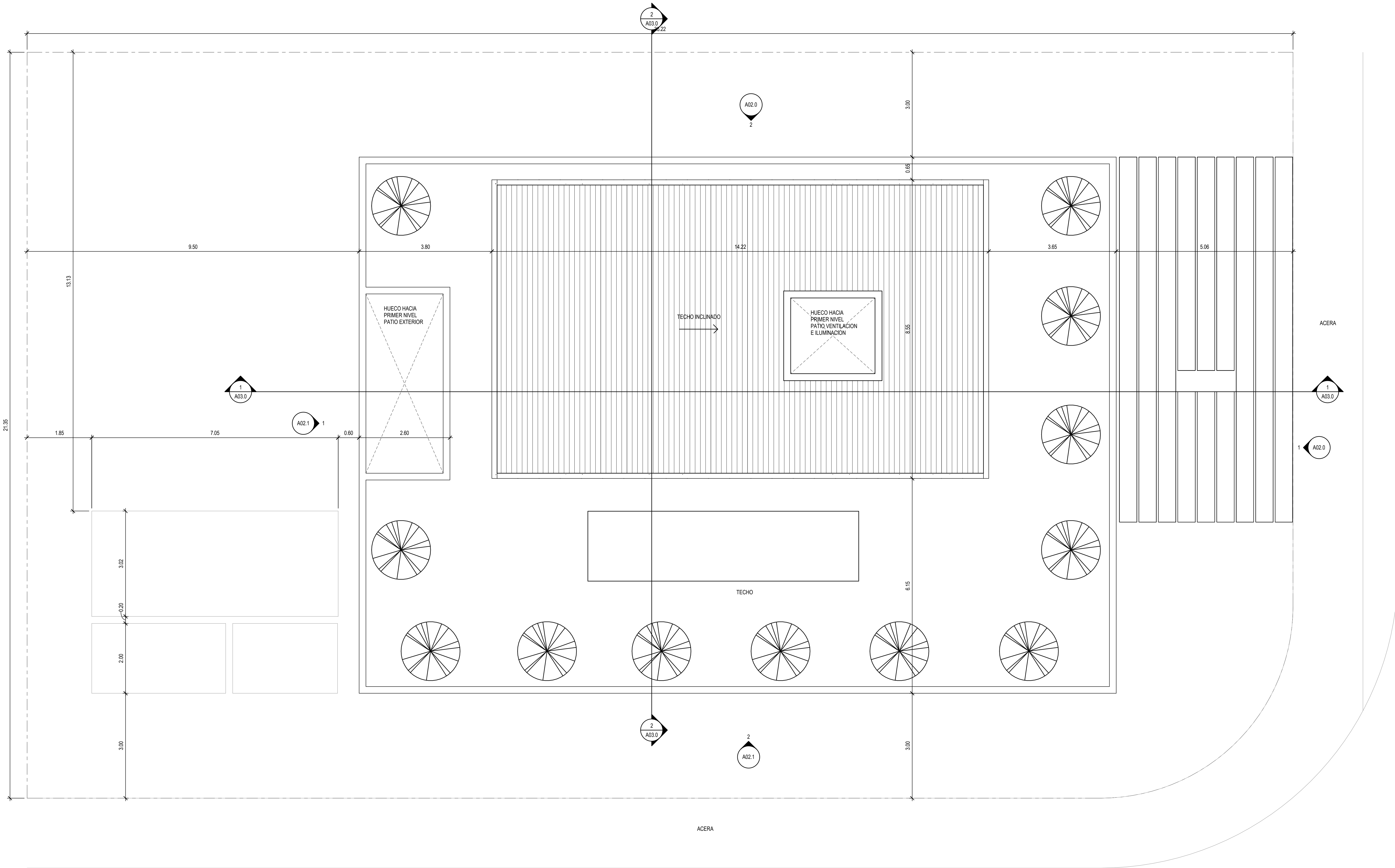
1 PLANTA DE CONJUNTO SCALE: 1 : 50
