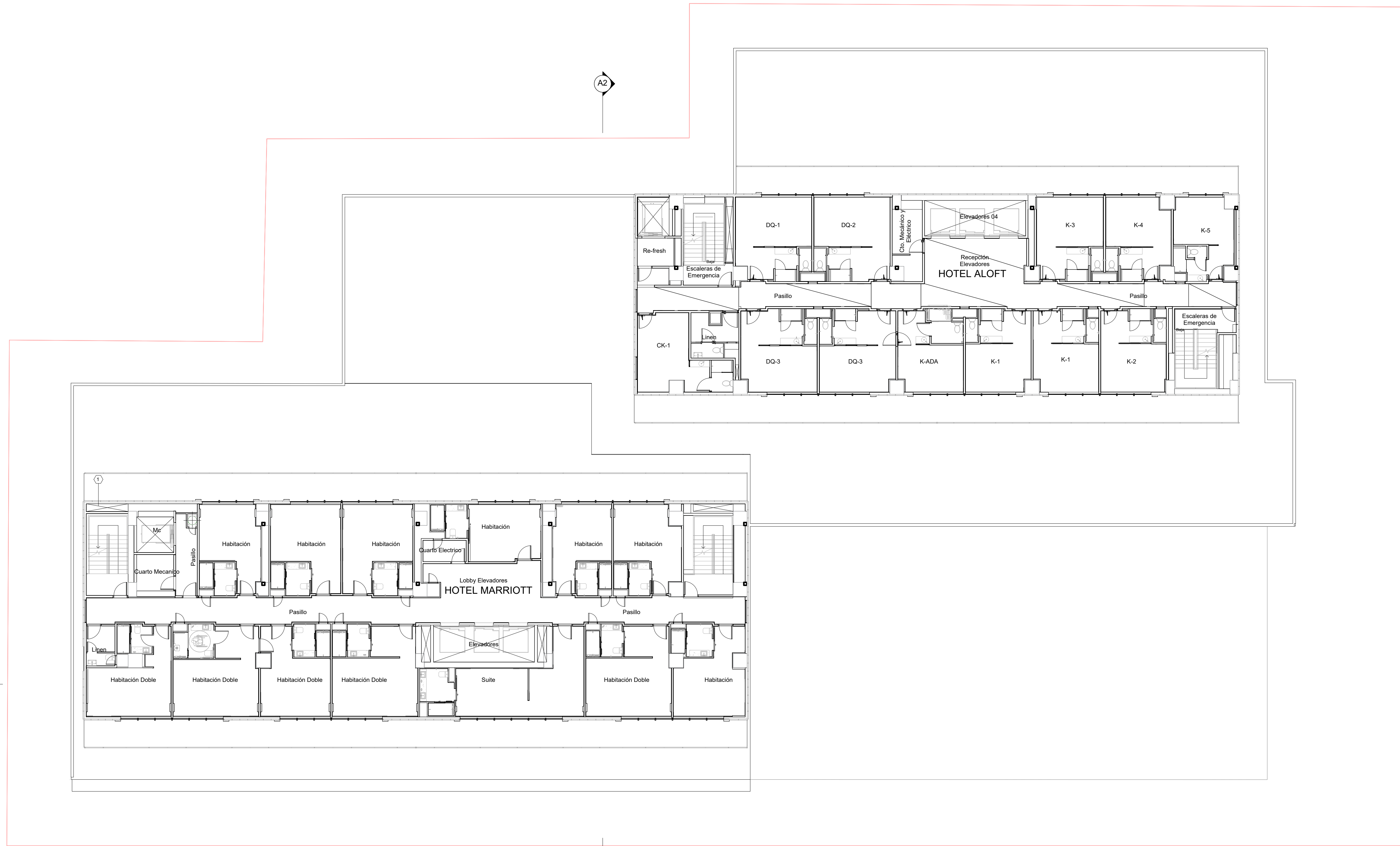
01 PLANTA ARQUITECTÓNICA NIVEL 4-19 1:150
