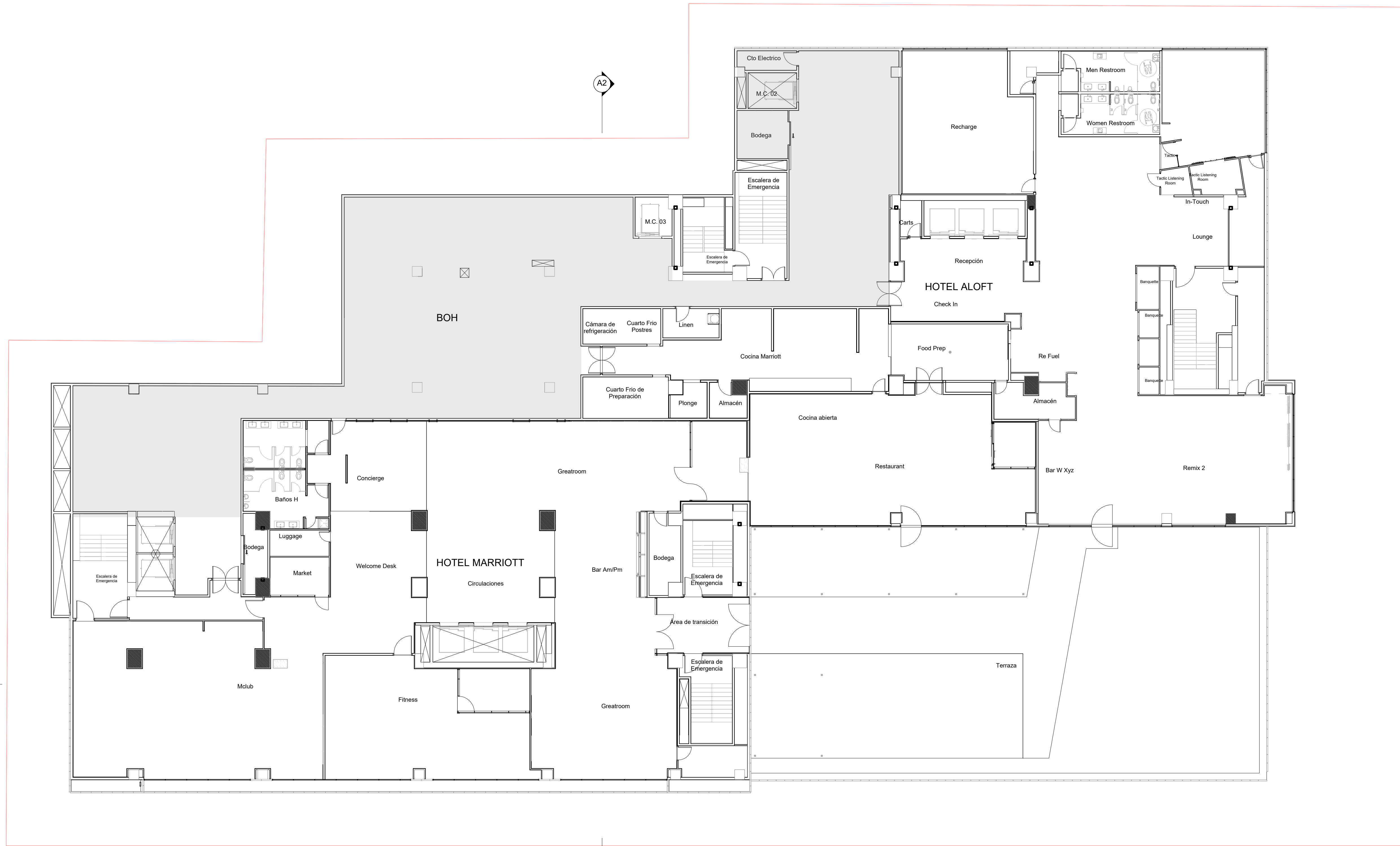
01 PLANTA ARQUITECTÓNICA 3ER NIVEL
