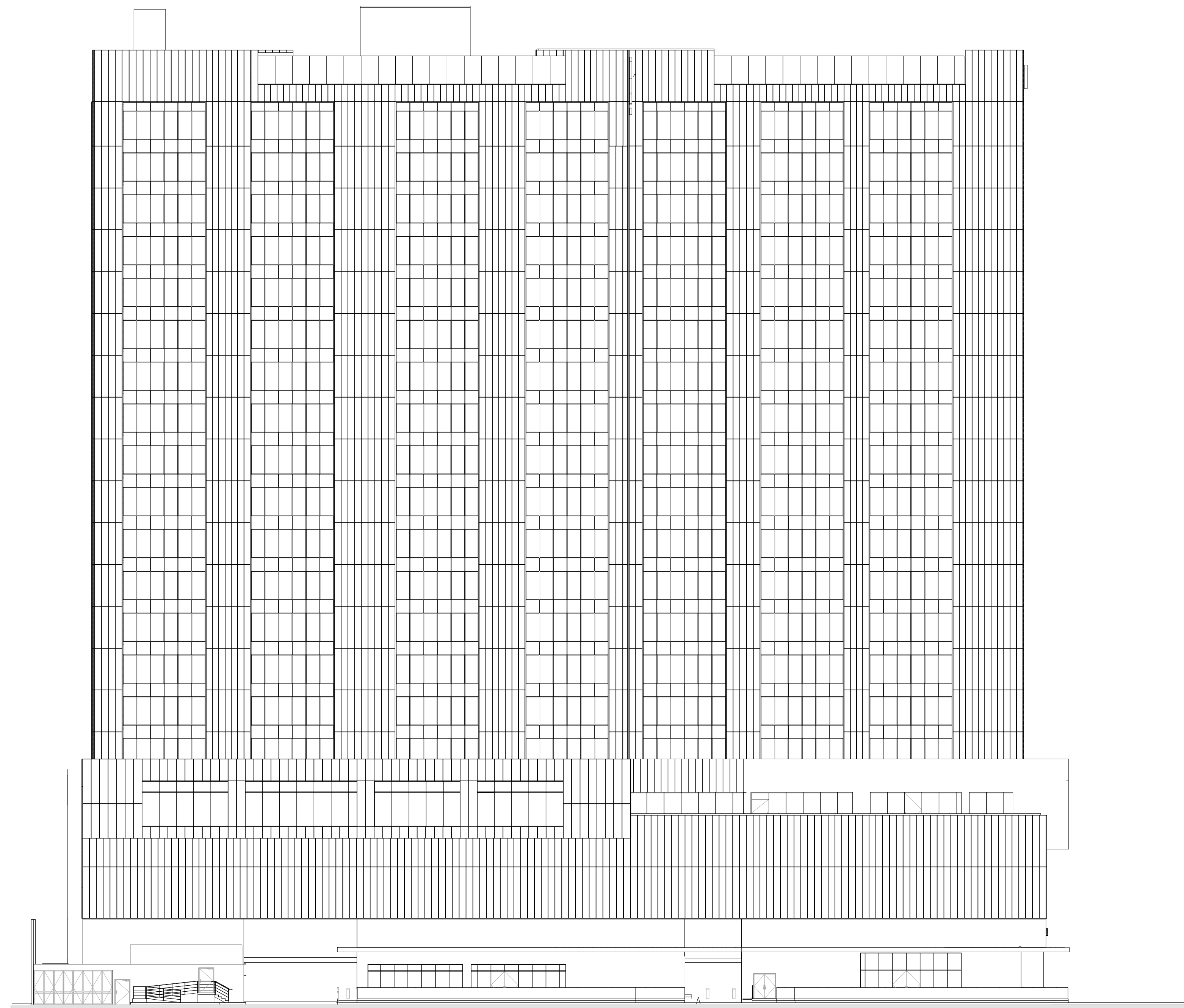
01 ELEVACIÓN NORTE 1:250
