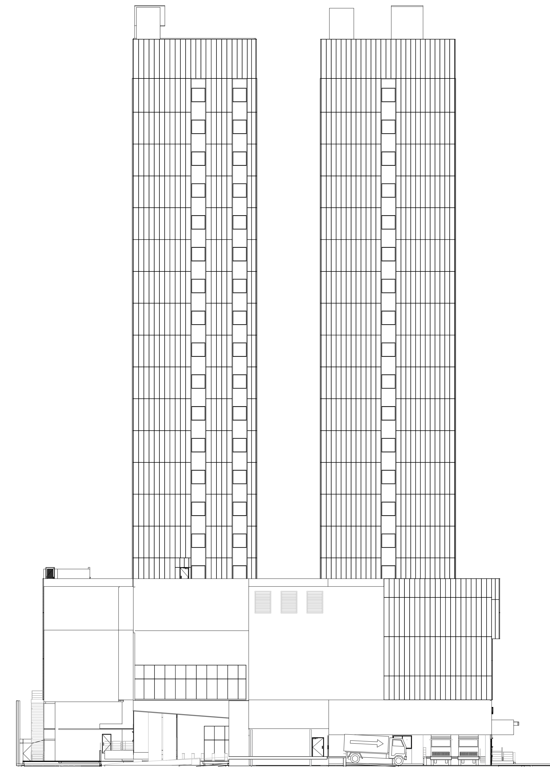
02 ELEVACIÓN ESTE 1:250
