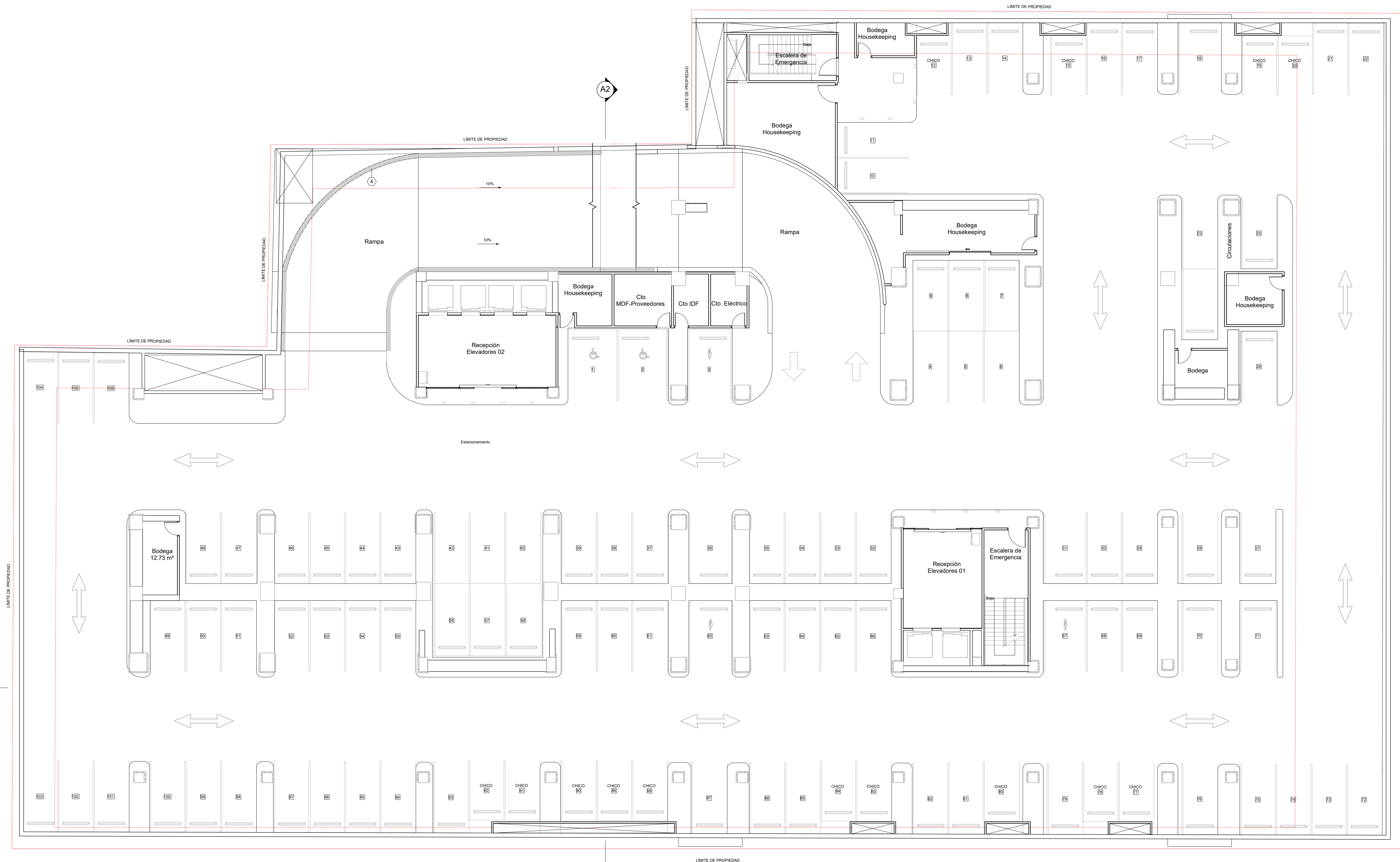
01 PLANTA SÓTANOS (TIPO) 1 : 150
