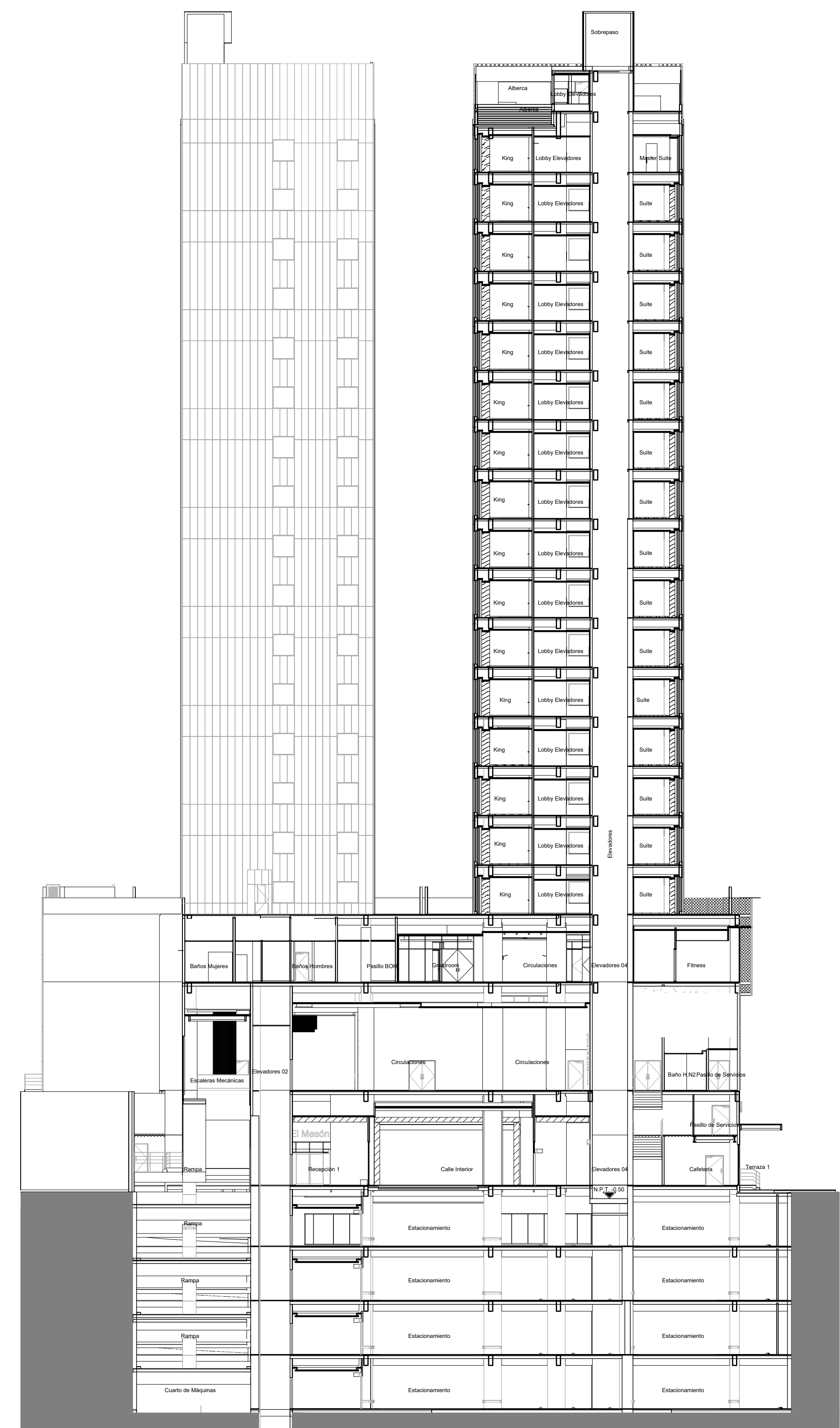
02 SECCIÓN A2 1 : 250
