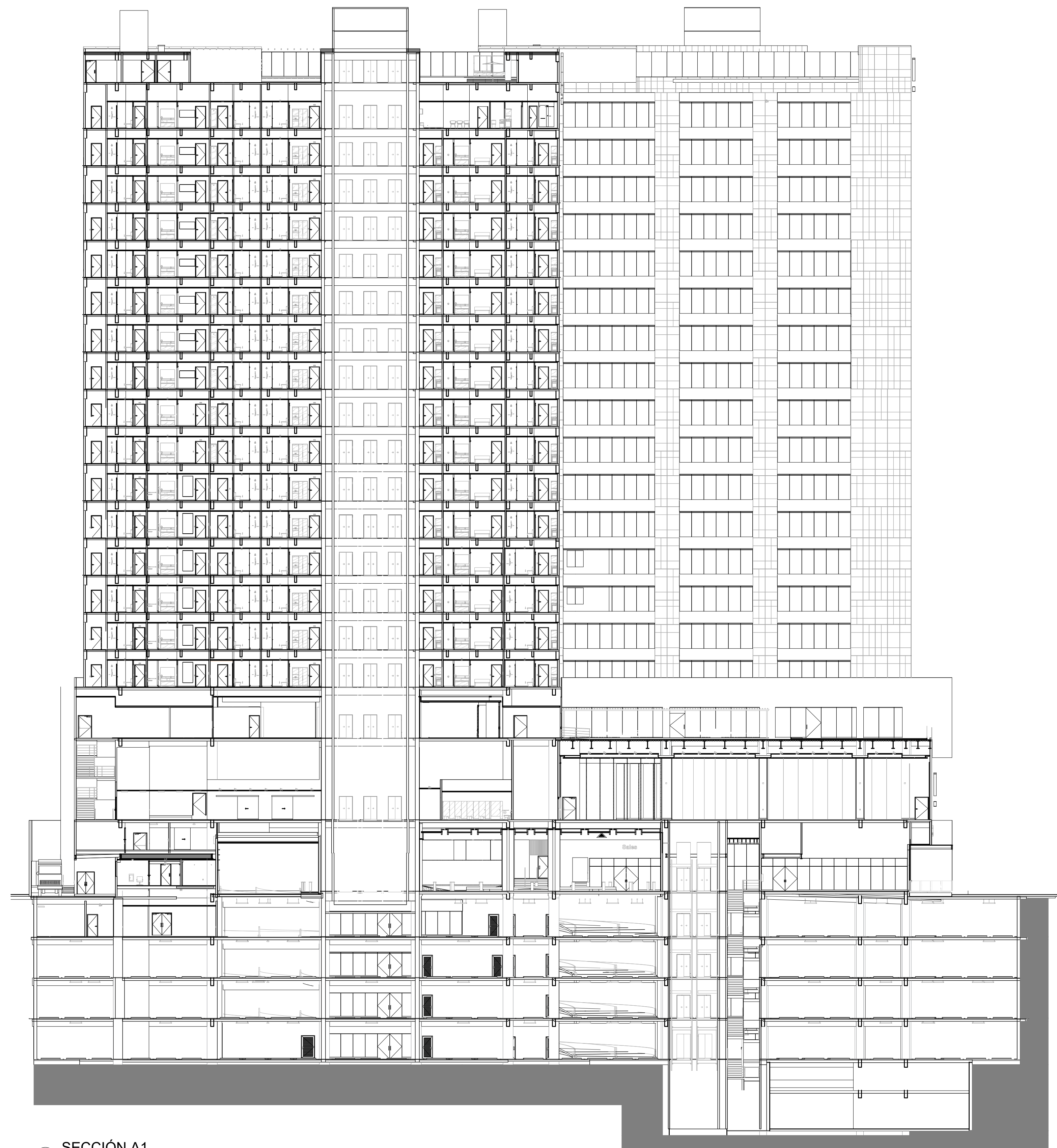
01 SECCIÓN A1 1 : 250
